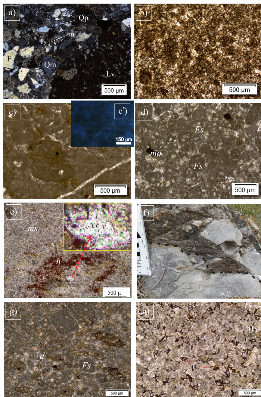
Figura 5. Petrografía de muestras en las formaciones Novillo y Olvido. a) Litarenita con granos de cuarzo monocrystalino (Qm), líticos volcánicos (Lv), cuarzo policristalino (Qp), feldespato (F), en matriz arcillosa (m), cemento calcáreo y minerales opacos, en el contacto transicional entre la Formación La Joya y la Formación Novillo (nicols cruzados); b) wackestone de peloides, arcilloso y dolomitizado; c) grainstone oncolítico, con epifluorescencia (c') hay contenido pobre de querógeno; d) caliza grainstone de ooides (cf. Favreina salivensis Fv) y minerales opacos (mo), cerca del contacto con la Formación Olvido; e) caliza mudstone (ms) con cristales de circón (cr) incluidos en vidrio (v) amorfo (en recuadro superior derecho) y hematita (h) luz natural, en el miembro medio de la Formación Olvido (muestra JP 125-03); f) Detalle de la superficie de erosión rellena por brecha en el contacto de las formaciones Olvido y La Casita; g) caliza grainstone de ooides (cf. Favreina salivensis Fs), parcialmente dolomitizada (d), con minerales opacos; h) macrolitolomía con porosidad intercrystalina (P).
