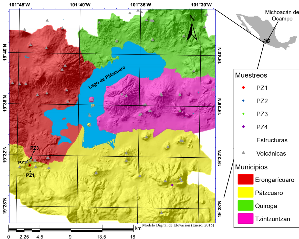
Figura 2. Modelo Digital de Elevación indicando los municipios cercanos al Lago de Pátzcuaro, distribución de los muestreos y estructuras de otros aparatos volcánicos.
