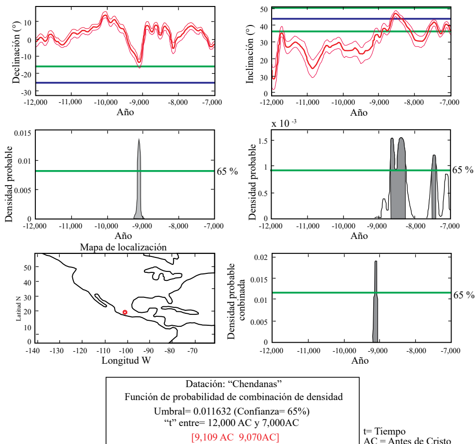
Figura 10. Gráficas de Declinación, Inclutación e Intensidad y edad para el flujo del Cerro Chendanas (circulo rojo en el mapa), dentro del recuadro se muestra en color rojo el intervalo de edad más probable.
