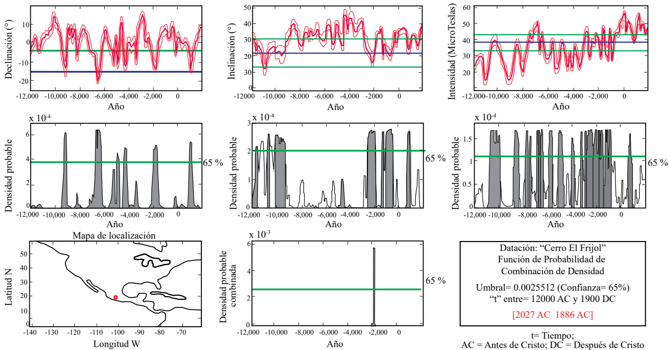
Figura 11. Gráficas de Declinación, Inclutación e Intensidad y edad para el flujo del Cerro El Frijol (circulo rojo en el mapa), dentro del recuadro se muestra en color rojo el intervalo de edad más probable.
