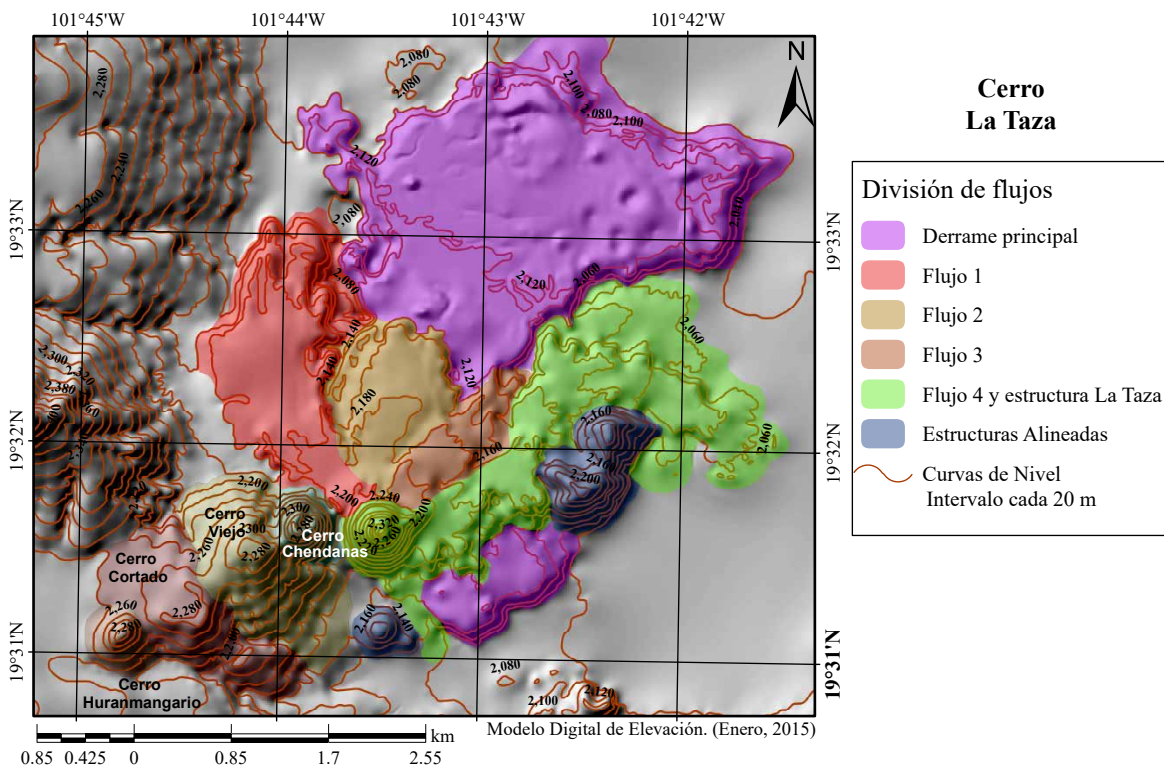
Figura 8. Detalle y división de flujos de lava del Cerro La Taza.
