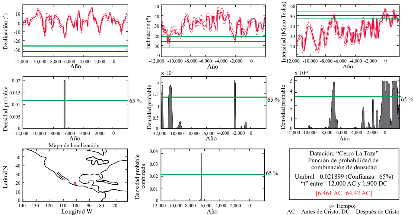
Figura 7. Gráficas de Declinación, Inclinación e Intensidad y edad para el flujo del Cerro La Taza (circulo rojo en el mapa), dentro del recuadro se muestra en color rojo el intervalo de edad más probable.
