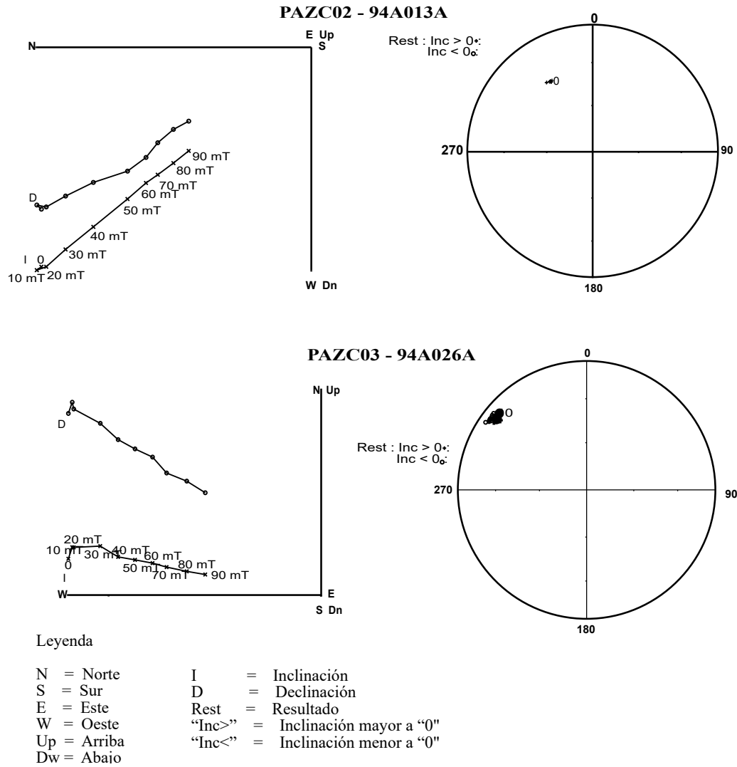
Figura 5. Ejemplos representativos de las curvas ortogonales (también conocidos como diagramas de Zijdeveld) obtenidas mediante desmagnetización por campos alternos. Nota: “Up”= parte superior, “Dn” = parte inferior. “Rest :Inc >, <” = son los resultados de las inclinaciones mayores o menores a “0”.
