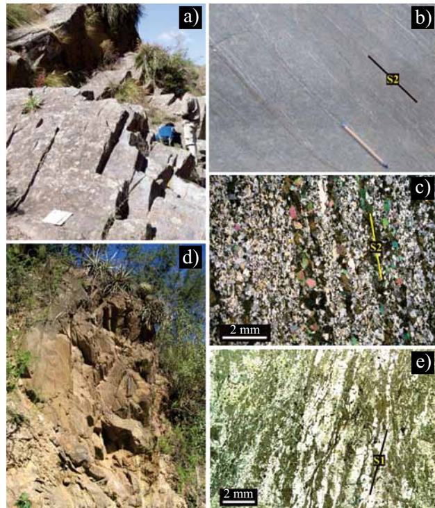
Figura 3. Fotografías de a) afloramiento; b) estructura mesoscópica; y c) mineralogía y microestructura, de los esquistos biotítico-muscovíticos del CMIEP; d) afloramiento de metasedimentos de bajo grado del CMLC; e) microestructura de las filitas del CMLC, se aprecia una alternancia de bandas lepidoblásticas ricas en clorita con bandas granoblásticas ricas en cuarzo y feldespatos.
