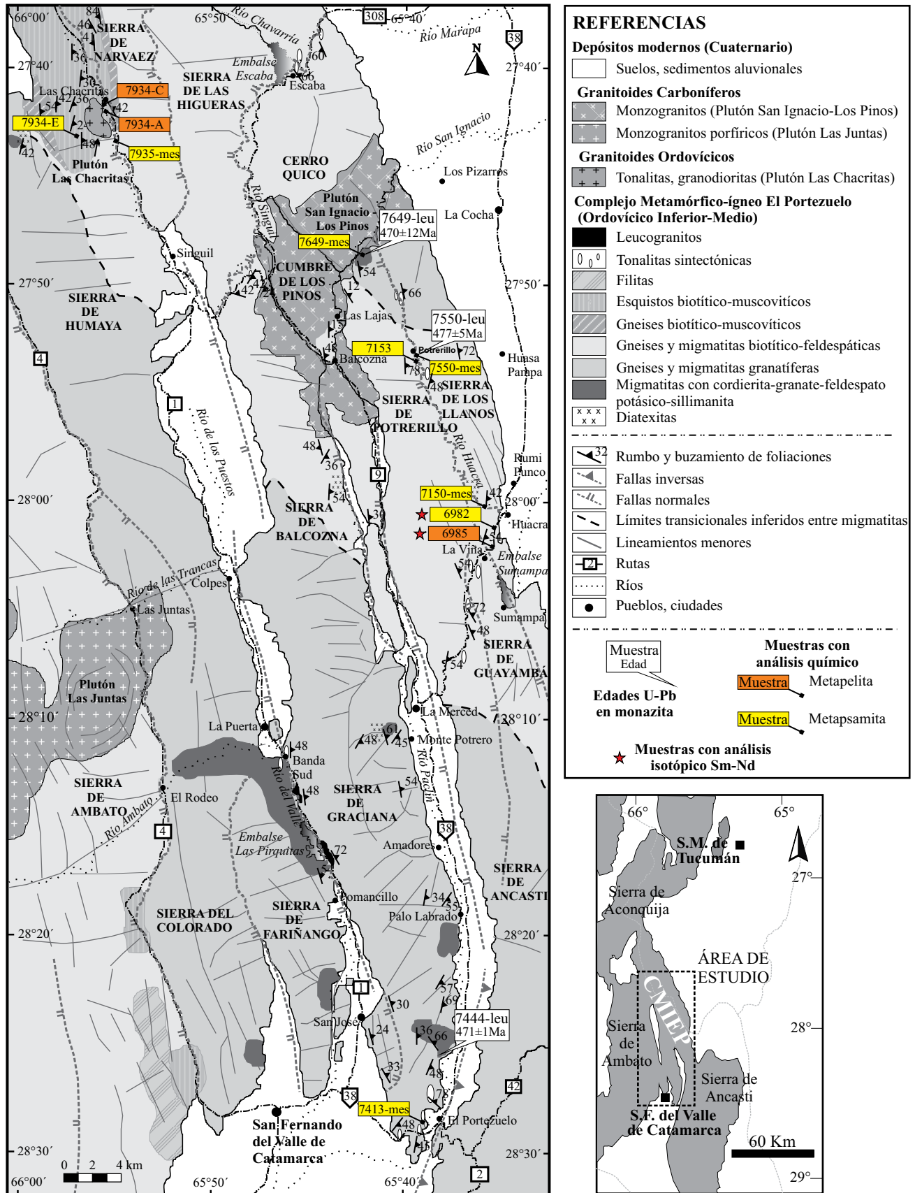
Figura 2. Mapa geológico del área de estudio en el sector nororiental de las Sierras Pampeanas en donde se indican las localidades muestreadas del complejo metamórfico-ígneo El Portezuelo. Interpretación de fallas según Gutiérrez y Mon (2008).
