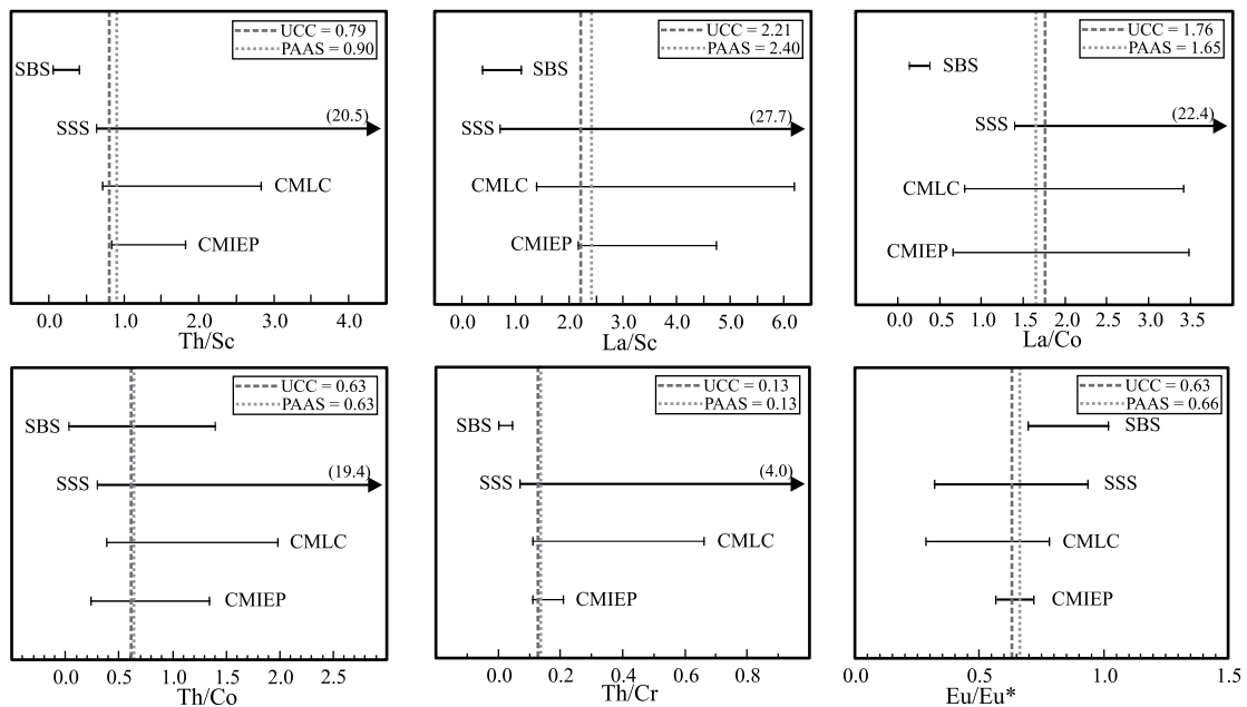
Figura 10. Comparación de las relaciones La/Sc, Th/Sc, La/Co, Th/Co, Th/Cr y Eu/Eu* entre el CMIEP y el CMLC, y con sedimentos provenientes de fuentes silíceas y de fuentes ígneas básicas determinadas por Cullers (2000). SSS (sediment from silicic sources): rango de sedimentos provenientes de fuentes ácidas; SBS (sediment from basic sources): rango de sedimentos provenientes de fuentes básicas. Como referencia también se muestran los valores de las relaciones de elementos de PAAS y UCC.
