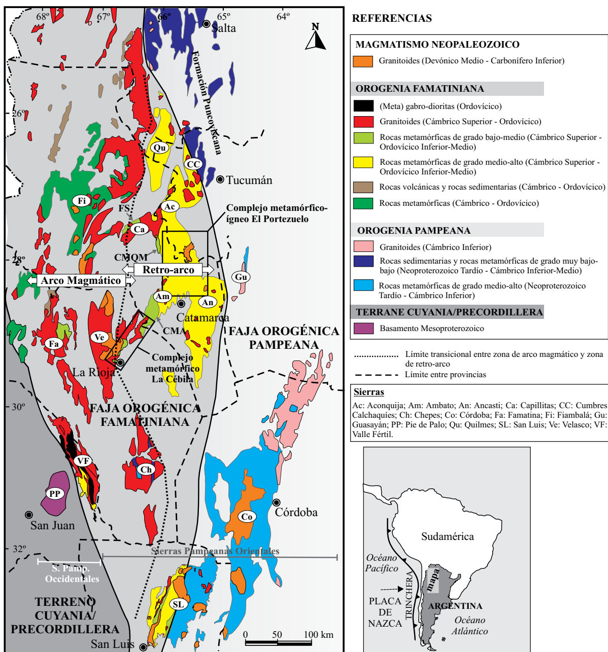
Figura 1. Mapa esquemático regional de las Sierras Pampeanas de Argentina mostrando la distribución relativa de las orogenias Pampeana y Famatiniana, las principales unidades litológicas y los complejos metamórficos Famatinianos. Modificado de Larrovere et al. (2011). CMQM: complejo metamórfico Quebrada del Molle; CMA: complejo metamórfico Ambato; FS: Formación Suncho.
