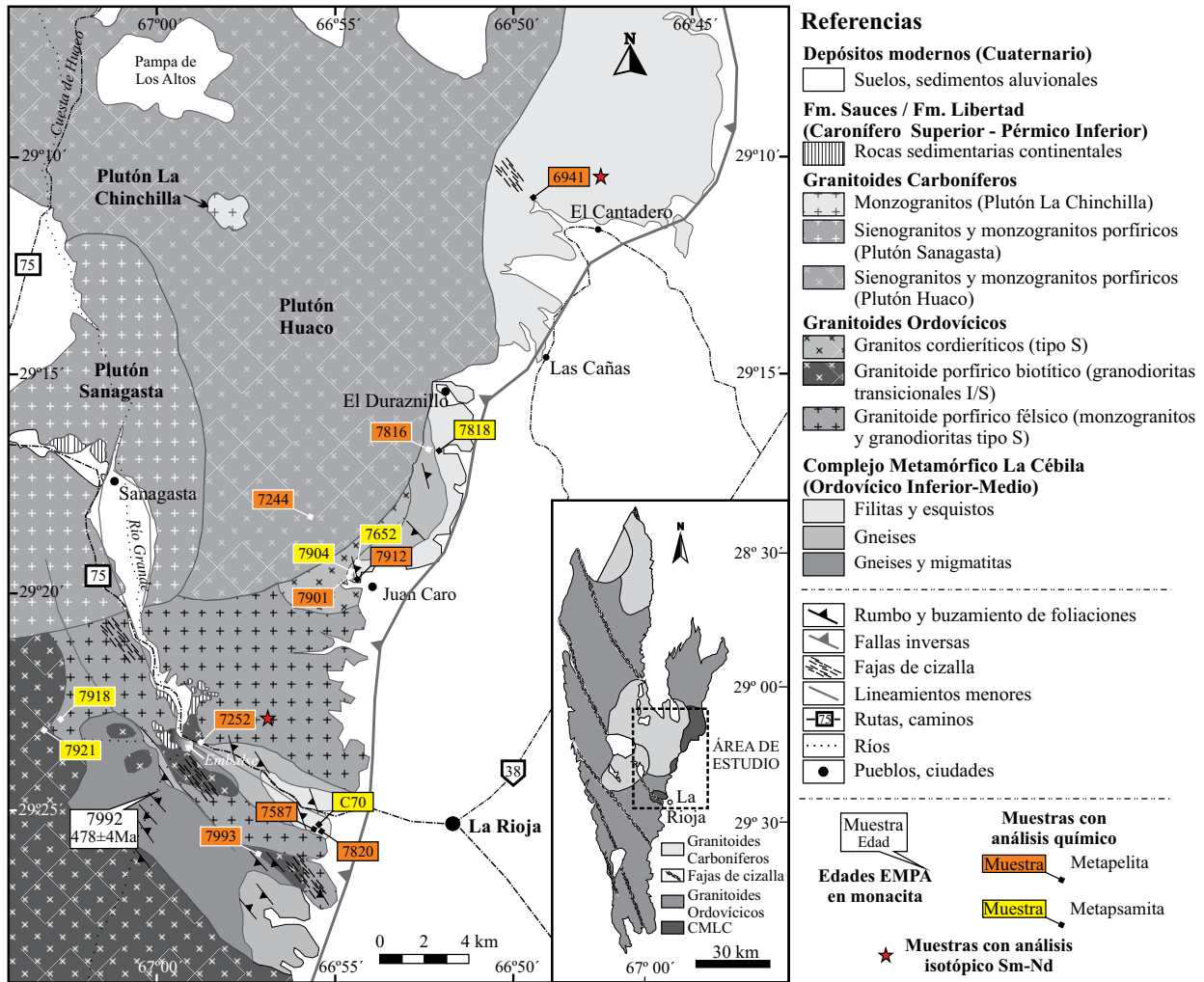
Figura 4. Mapa geológico del área de estudio en el flanco centro-oriental de la Sierra de Velasco en donde se indican las localidades muestreadas del complejo metamórfico La Cébila.
